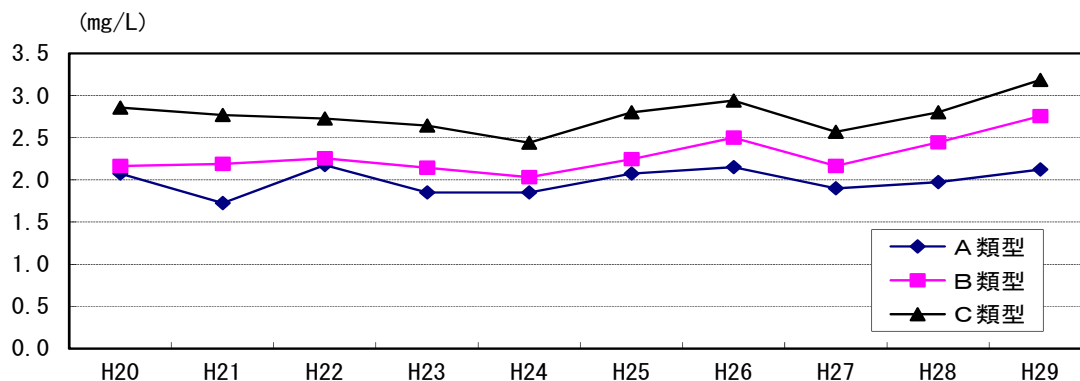
図 5 東京湾の化学的酸素要求量（COD）の濃度の推移（類型別の年平均値）
