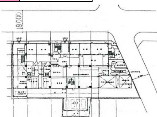
配置及び1階平面図
