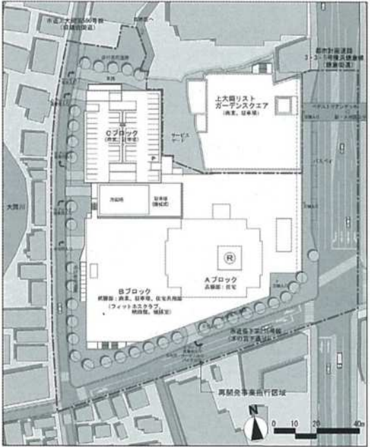
配置計画図
