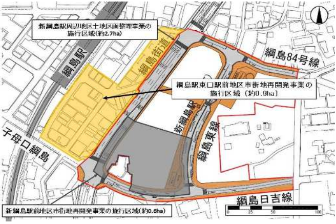
区域図
