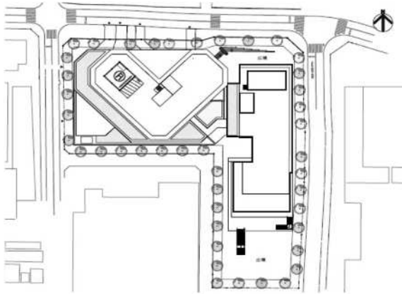
配置図
