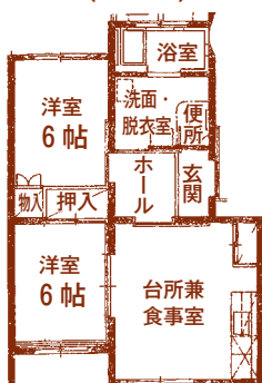
身体障害者向住宅 KF-6身(車いす単身) (2DK)
