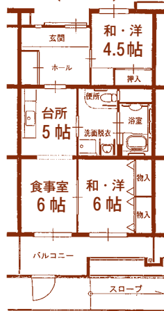
身体障害者向住宅 KF-6身(車いす単身) (2DK)
