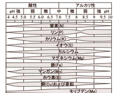
■ [図-2] 土壌pHと養分の溶解、利用度(Truog)
