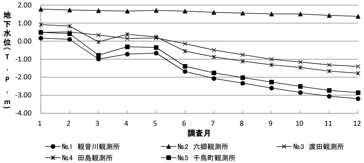
図7-7 平成30年地下水位の経月変化 (川崎市川崎区)
