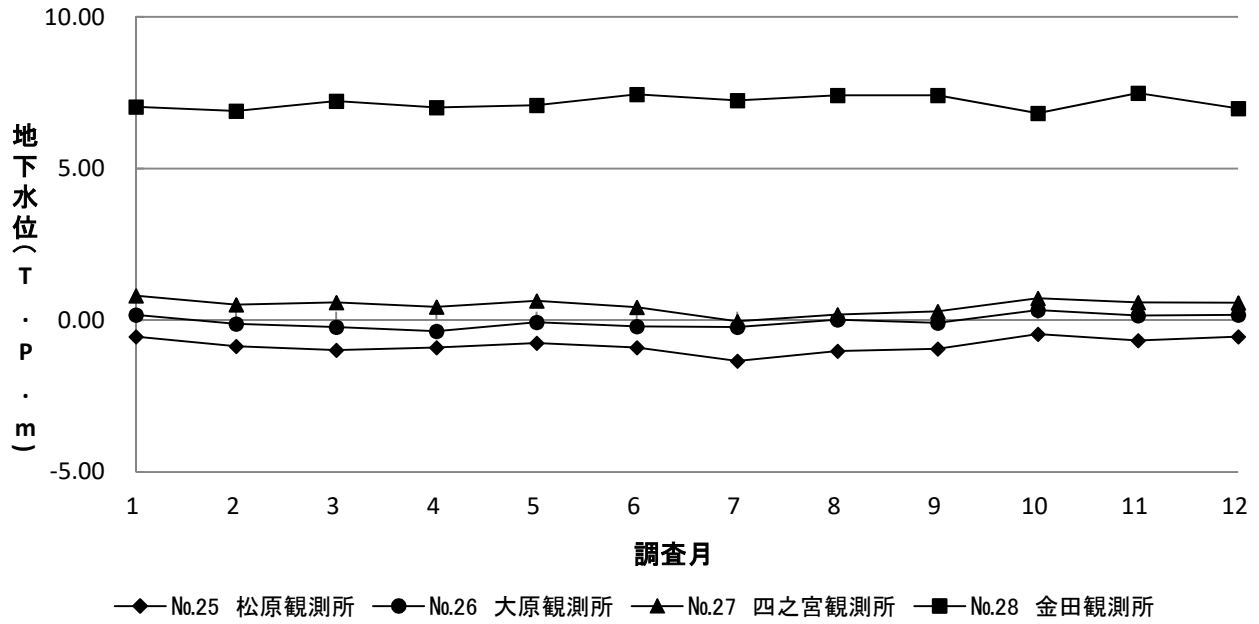
図7-9 平成30年地下水位の経月変化(平塚市)
