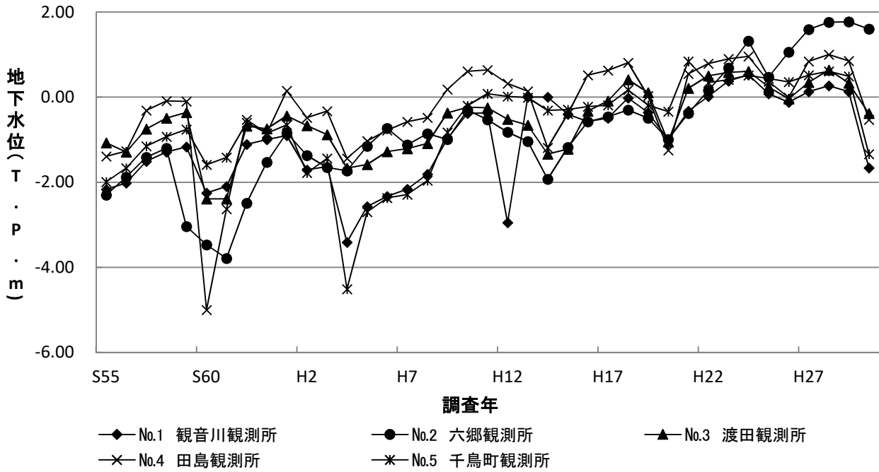
図7-1 地下水位の経年変化(川崎市川崎区)
