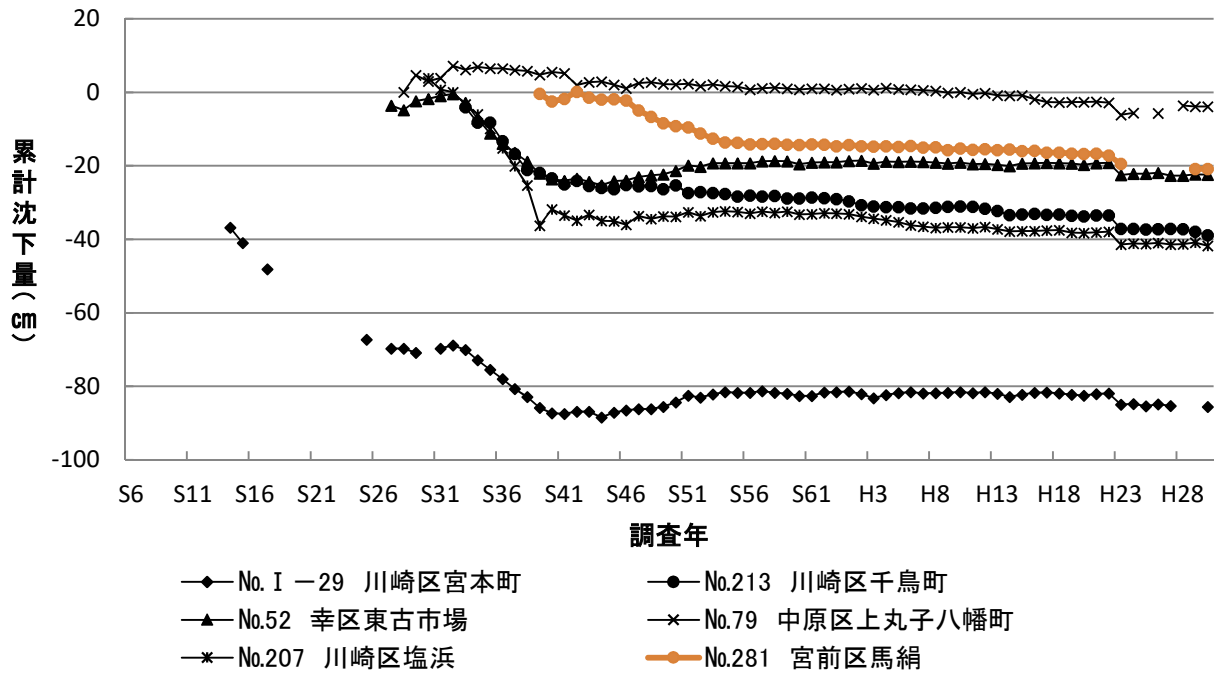
図4 主要水準点の沈下状況の経年変化 川崎地域
