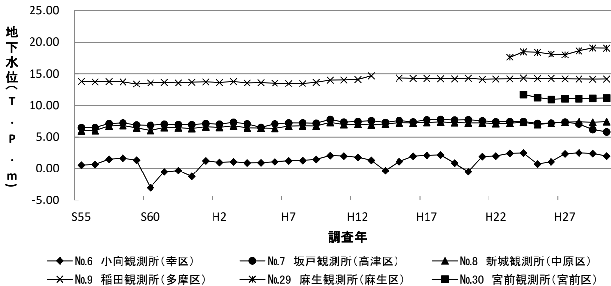
図7-2 地下水位の経年変化(川崎市幸区、高津区、中原区、多摩区、麻生区、宮前区)
