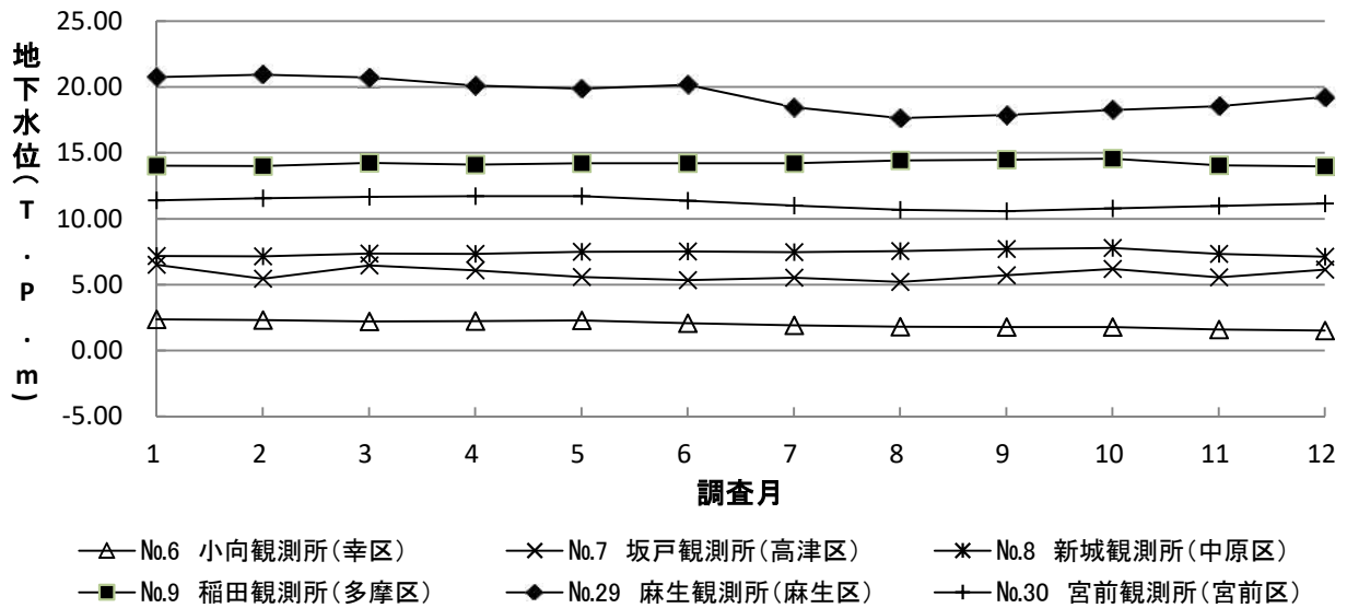
図7-8 平成30年地下水位の経月変化 (川崎市幸、高津、中原、多摩、麻生、宮前区)
