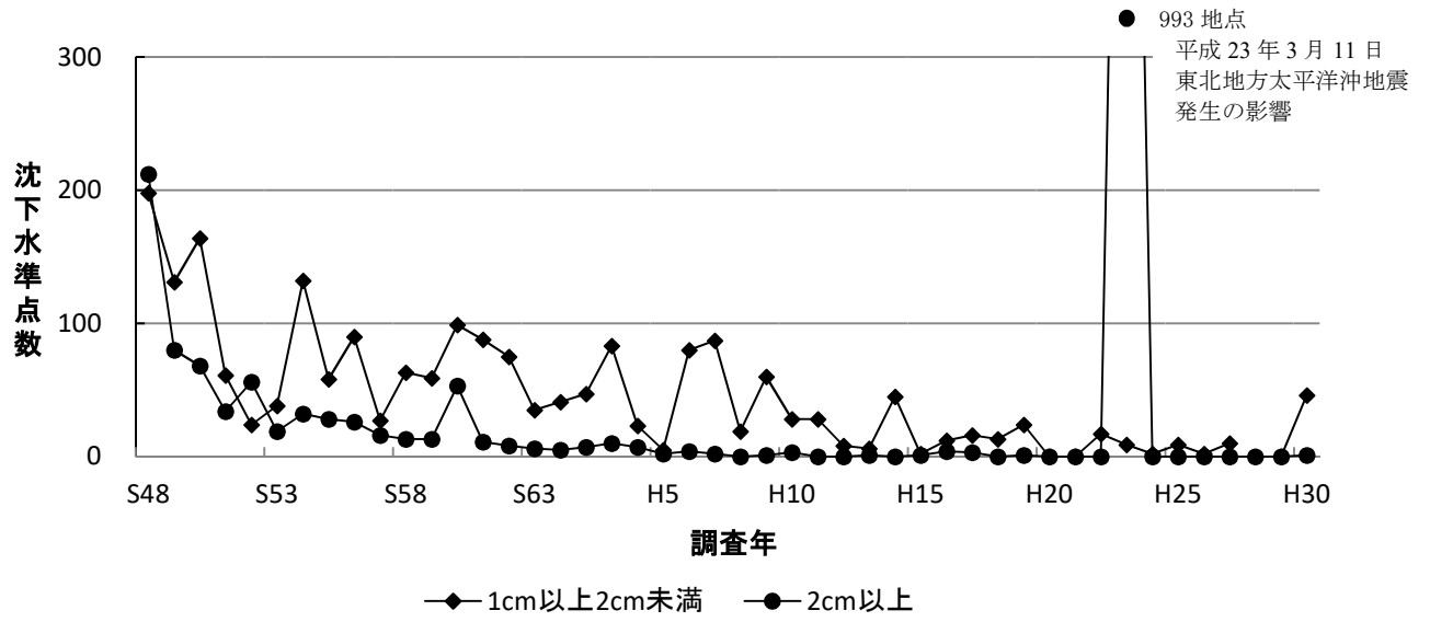
図2-1 1cm以上沈下水準点数の経年変化(全域)
