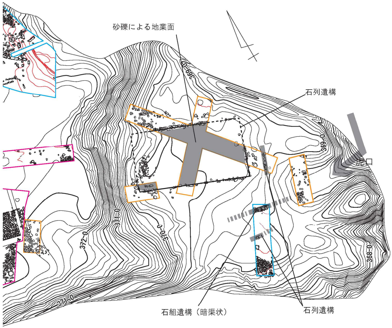
「土蔵」曲輪平面図
