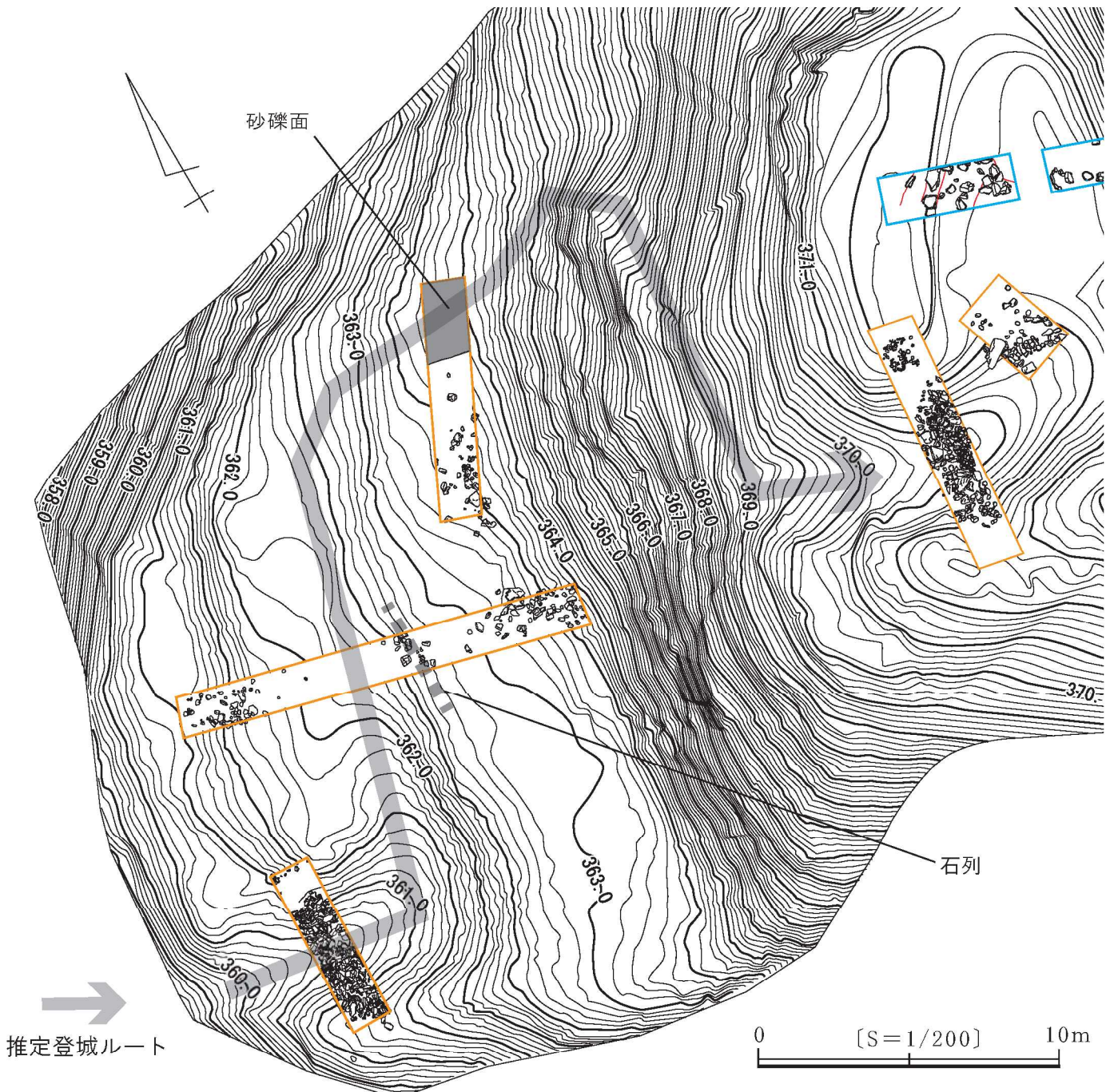
「米蔵」曲輪平面図
