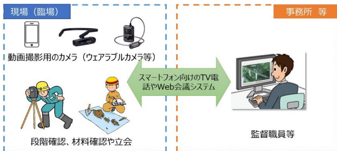
図 2-1 機器構成（例）
